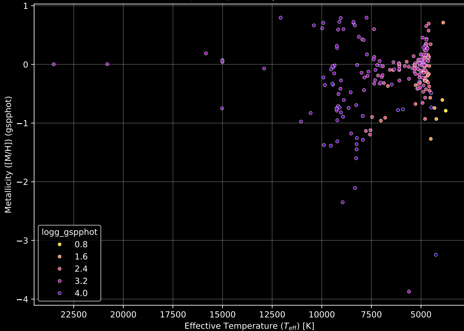
APOGEE DR17 Field: [296+00] Stellar Population Parameters (n= 227)
